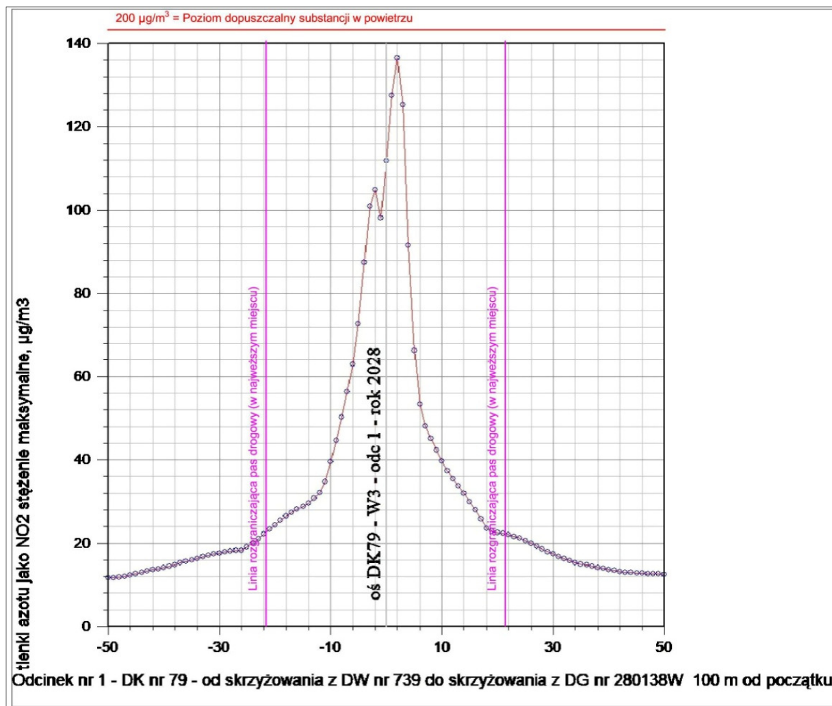
Rysunek 19. Rozkład maksymalnych stężeń jednogodzinnych S1 tlenków azotu jako dwutlenek azotu w przekroju poprzecznym (prostopadłym do osi drogi) rozbudowywanej drogi DK79 – odcinek nr 1 (DW739 ÷ DG nr 280138W) – rok 2028 – warianty W1, W2 i W3
