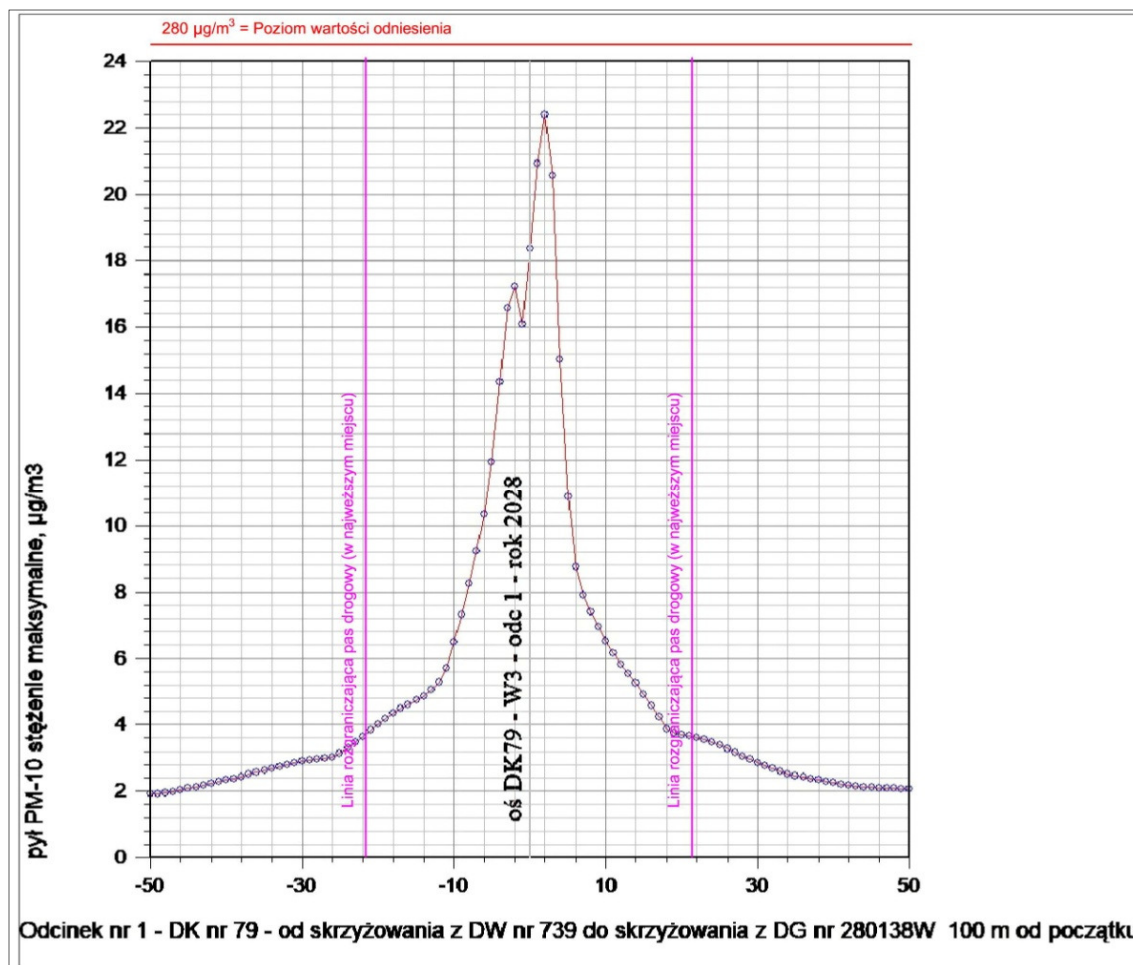
Rysunek 21. Rozkład maksymalnych stężeń jednogodzinnych S_1 pyłów zawieszonych PM10 w przekroju poprzecznym (prostopadłym do osi drogi) rozbudowywanej drogi DK79 – odcinek nr 1 (DW739 ÷ DG nr 280138W) – rok 2028 – warianty W1, W2 i W3
