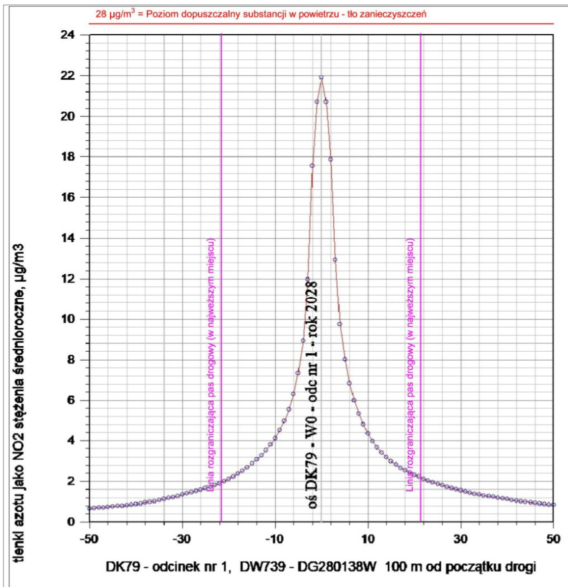
Rysunek 16. Rozkład stężeń średniorocznych S_a tlenków azotu jako dwutlenek azotu w przekroju poprzecznym (prostopadłym do osi drogi) rozbudowywanej drogi DK79 – odcinek nr 1 (DW739 ÷ DG nr 280138W) – rok 2028 – wariant W0
