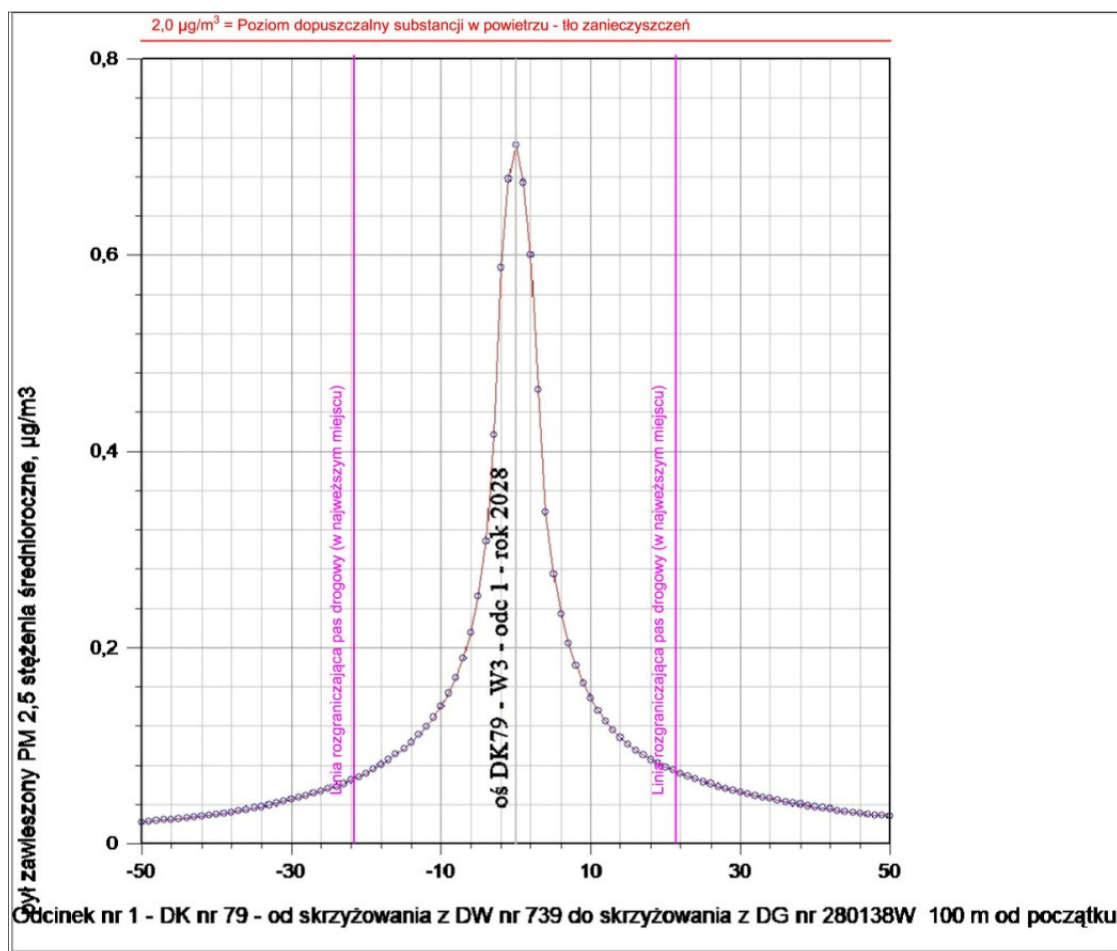
Rysunek 22. Rozkład stężeń średniorocznych S_a pyłów zawieszonych PM 2,5 w przekroju poprzecznym (prostopadłym do osi drogi) rozbudowywanej drogi DK79 – odcinek nr 1 (DW739 ÷ DG nr 280138W) – rok 2028 – warianty W1, W2 i W3
