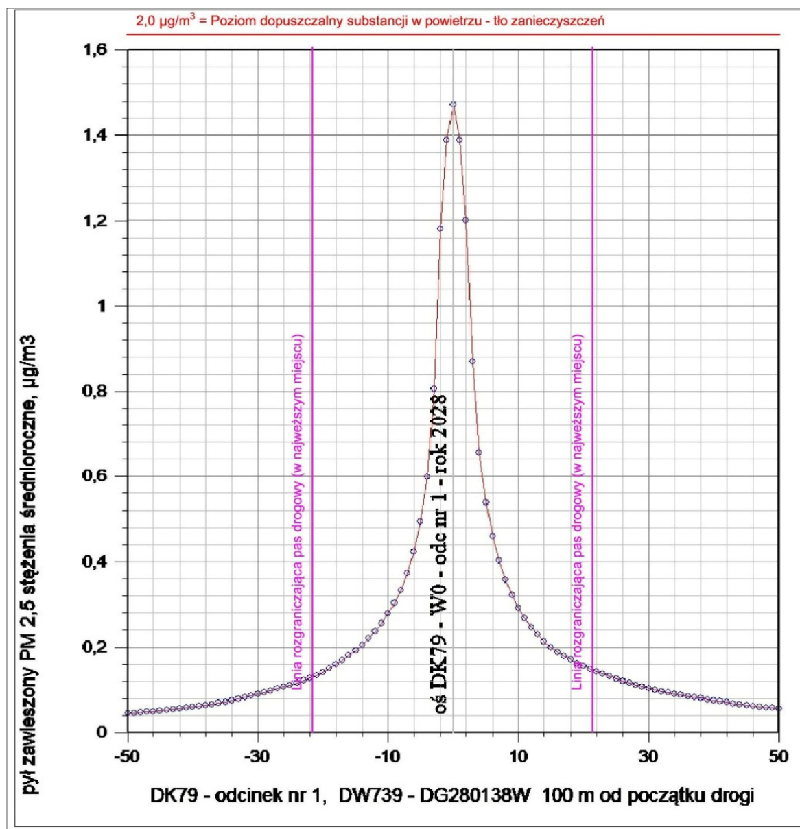
Rysunek 18. Rozkład stężeń średniorocznych S_a pyłów zawieszonych PM 2,5 w przekroju poprzecznym (prostym do osi drogi) rozbudowywanej drogi DK79 – odcinek nr 1 (DW739 ÷ DG nr 280138W) – rok 2028 – wariant W0
