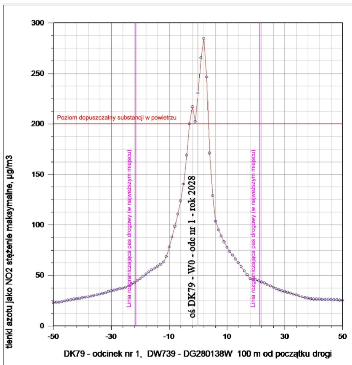
Rysunek 15. Rozkład maksymalnych stężeń jednogodzinnych S1 tlenków azotu jako dwutlenek azotu w przekroju poprzecznym (prostopadłym do osi drogi) rozbudowywanej drogi DK79 – odcinek nr 1 (DW739 ÷ DG nr 280138W) – rok 2028 – wariant W0
